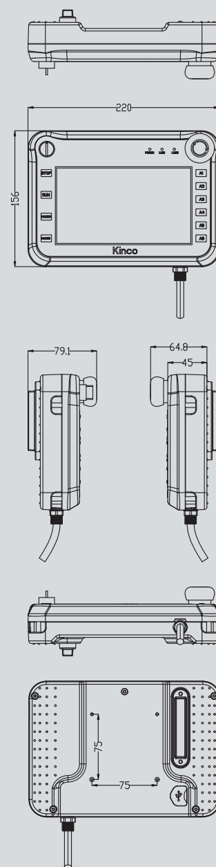
机械尺寸图 单位: mm
